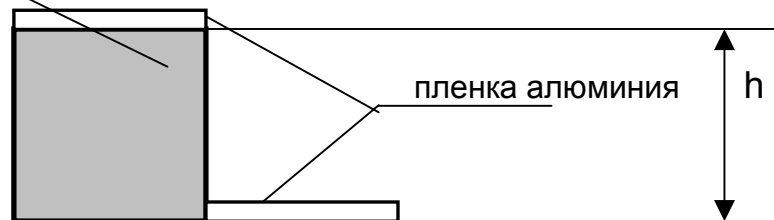
Рис.3. Измерение толщины пленки на микроинтерферометре МИИ-4.
